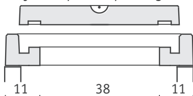
Tampon hydraulique N°3 pour regard 50 x 50
