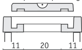
Tampon hydraulique N°1 pour regard 33 x 33
