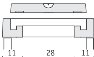
Tampon hydraulique N°2 pour regard 40 x 40
