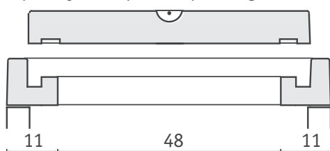
Tampon hydraulique N°4 pour regard 60 x 60
