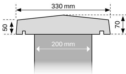
COUVERTINE 2 PENTES - MUR DE 20 cm
