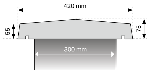
COUVERTINE 2 PENTES - MUR DE 30 CM
