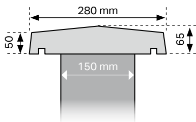
COUVERTINE 2 PENTES - MUR DE 15 cm
