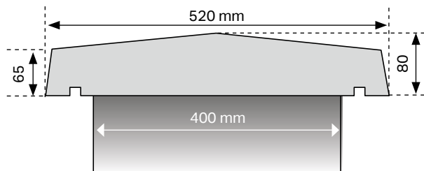
COUVERTINE 2 PENTES - MUR DE 40 CM
